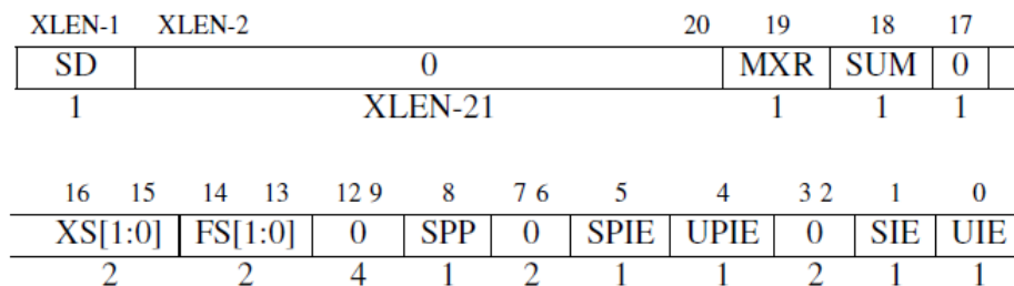
图 10.9: sstatus CSR。sstatus 是 mstatus（图 10.4）的一个子集，因此它们的布局类似。SIE 和 SPIE 中分别保存了当前的和异常发生之前的中断使能，类似于 mstatus 中的 MIE 和 MPIE。RV32 的 XLEN 为 32，RV64 为 40。（来自 [Waterman and Asanovic 2017] 中的图 4.2；有关其他域的说明请参见该文档的第 4.1 节。）
