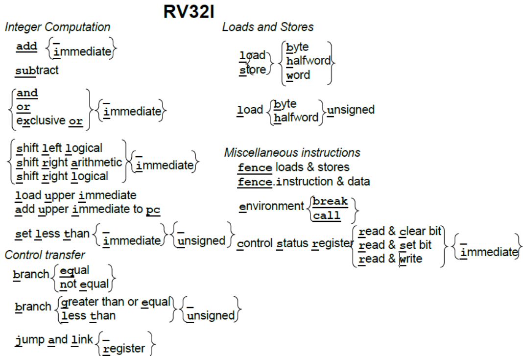
图 2.1: RV32I 指令图示。把带下划线的字母从左到右连接就组成了 RV32I 指令。花括号 {} 表示集中垂直方向上的每个项目都是指令的不同变体。集合中的下划线_意味着不包含这个字母的也是一个指令名称。例如，左上角附近的符号表示以下六个指令：and, or, xor, andi, ori, xori。
